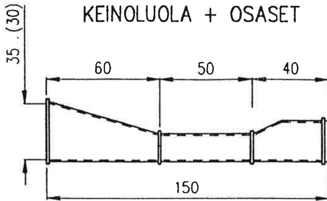
AHDINKOPUTKI, SIVUPROFIILI
